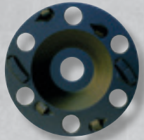
PNC125-803-B2 Plateau ø 125 mm 2 segments 5,5 mm 4 polycristallins en arrondi
