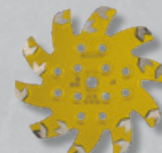
PN255-F15 Plateau ø 250 mm 15 segments flèches
