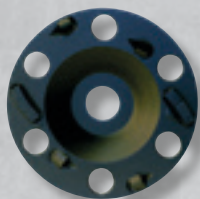
PNC125-803-B2 Plateau ø 125 mm 2 segments 5,5 mm 4 polycristallins en arrondi
