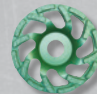
PNG125 Plateau ø 125 mm 16 segments H.5,5 mm
