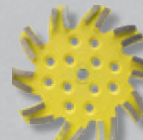
PN255-E20 Plateau ø 250 mm 20 segments H.10 mm Spécial dégrossissage
